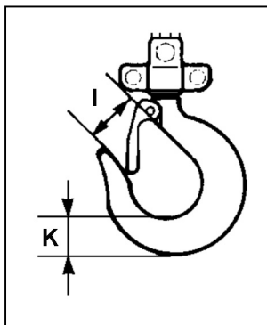
Fig 4 Lastkrok
