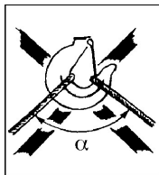
Fig. 2 b For stor toppvinkel på slyngen!
