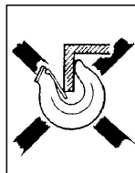
Kuva 2 d Koukun kärkeen vaikuttaa lisäksi vääntävä kosketusrasitus!
