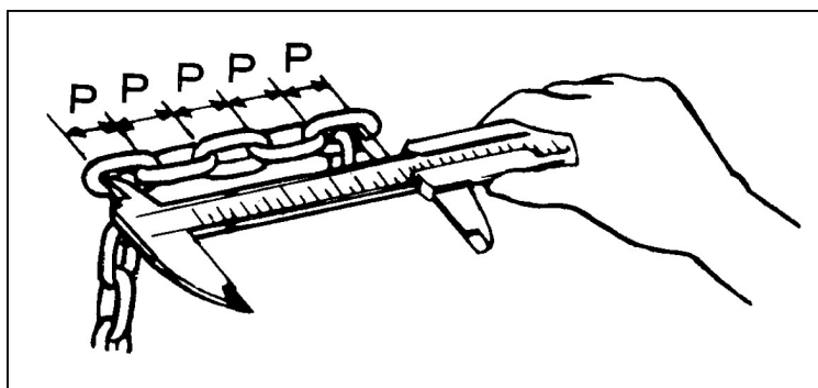
Kuva 5 Kuormaketjun kontrollimittaus
