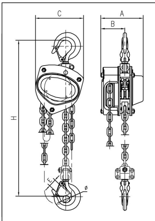
Fig 1 Måttskiss
